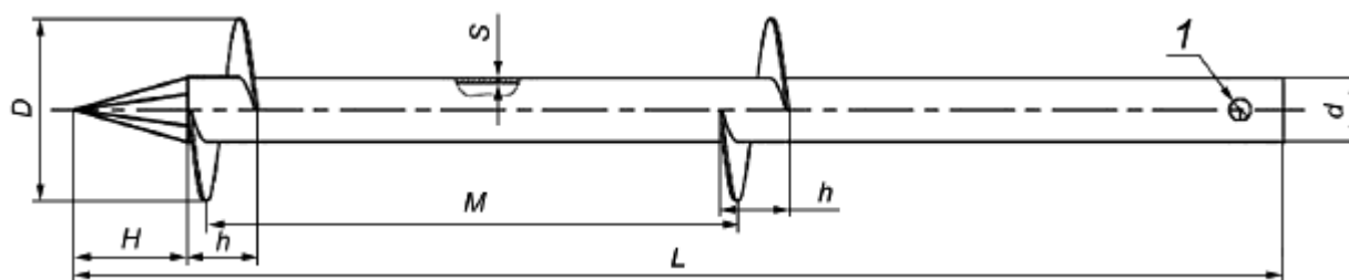
в - свая винтовая двухлопастная
