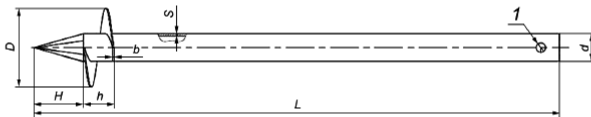
а - свая винтовая лопастная
